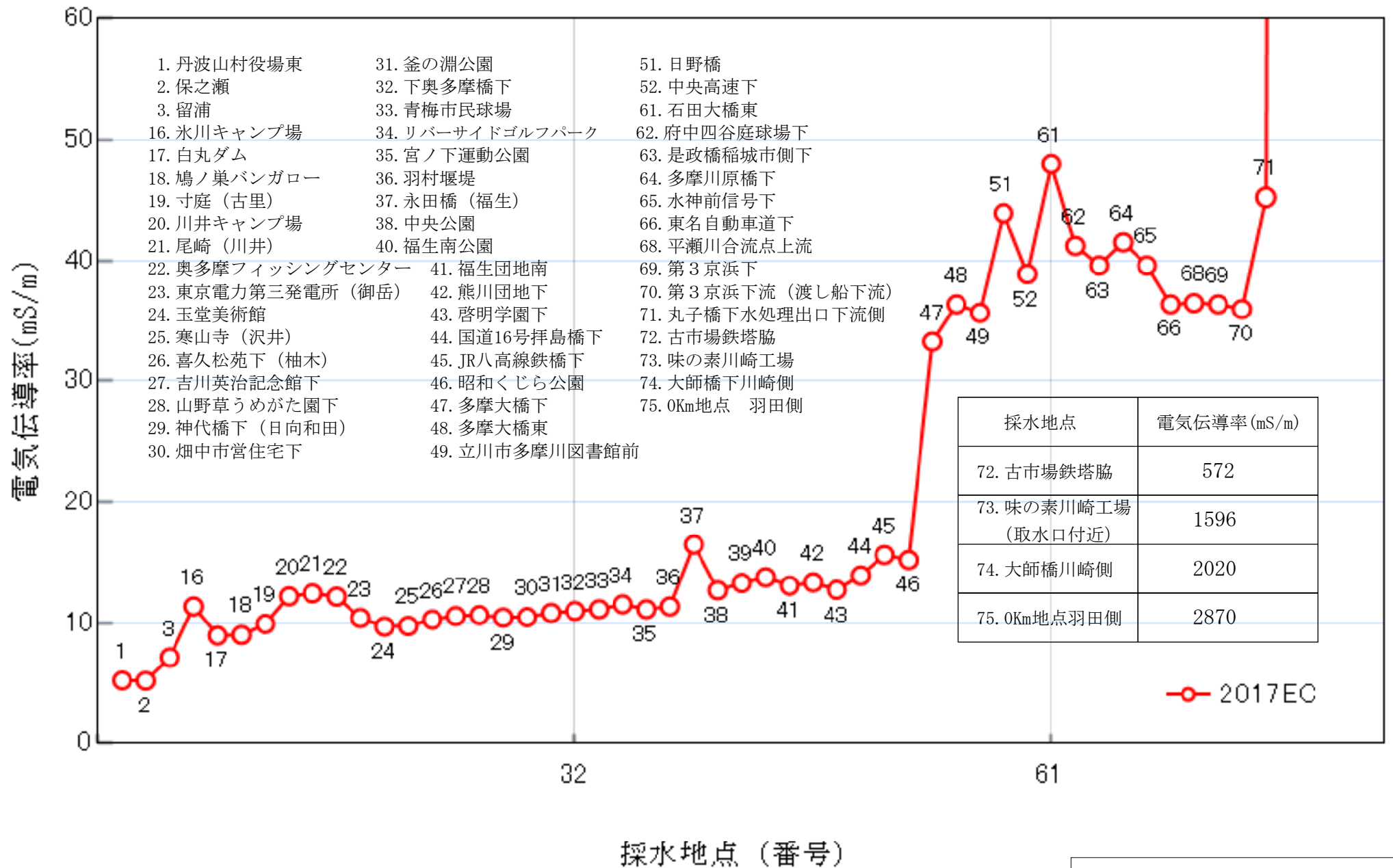
図1 多摩川本川の電気伝導率 (2017.6.4)
