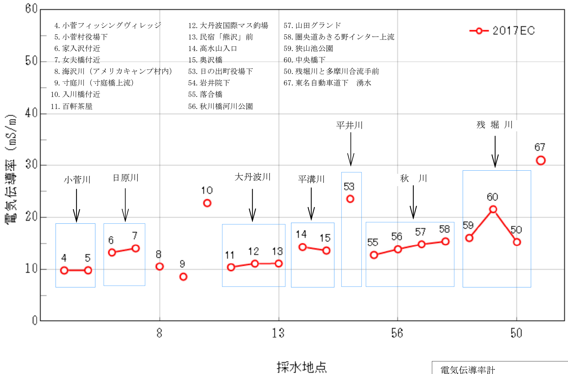
図2 多摩川支川の電気伝導率 (2017.6.4)
