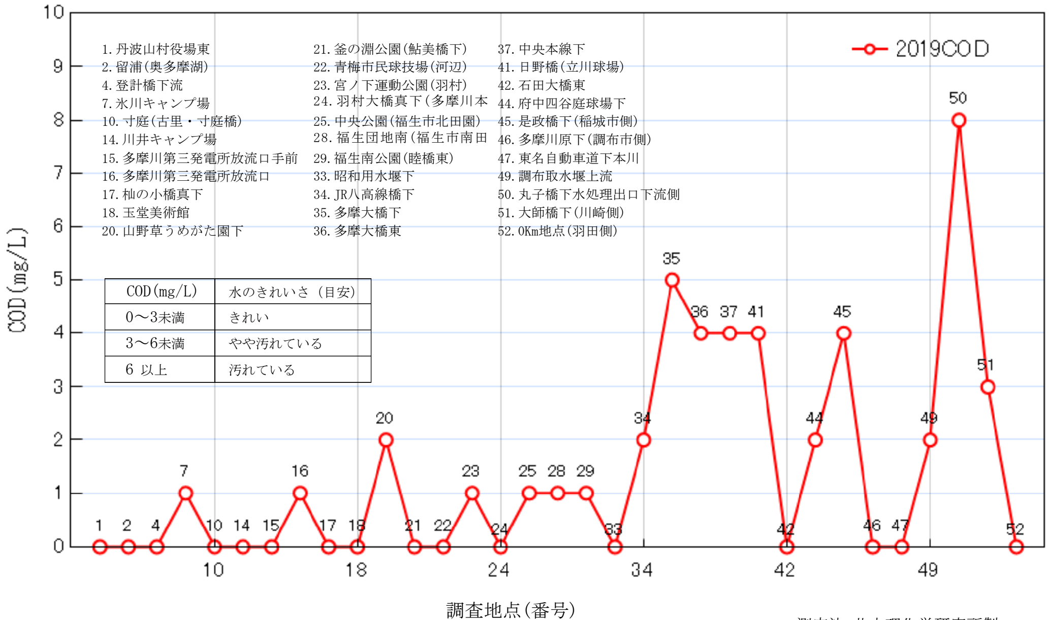
多摩川本川のCOD(2019. 6. 2)
